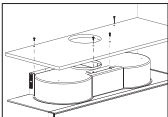
層板安裝
