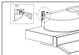
壁掛式安裝
