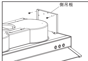
側吊板安裝*
