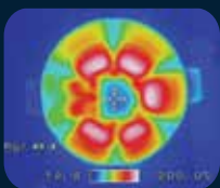
一般單環外焰火 高溫區面積 275cm 2
